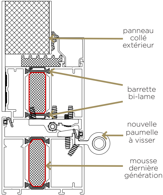
Version 2 Panneau collé extérieur
