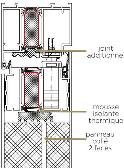
Version 3 Panneaux collés 2 faces
