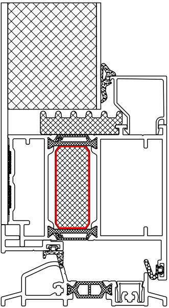
Seuil PMR porte ouverture intérieure - panneau collé 1 face
