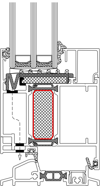
Seuil PMR porte ouverture ext/int - triple vitrage
