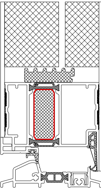
Seuil PMR porte ouverture intérieure - panneau collé 2 faces
