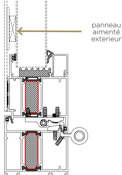
Version 4 Panneau aimenté extérieur
